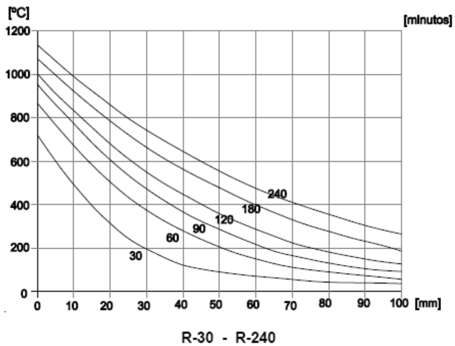
Figura C.8. Distribución de temperaturas en el espesor de secciones planas expuestas por una cara h \geq 200
