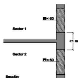
Figura 1.7 Encuentro forjado-fachada
