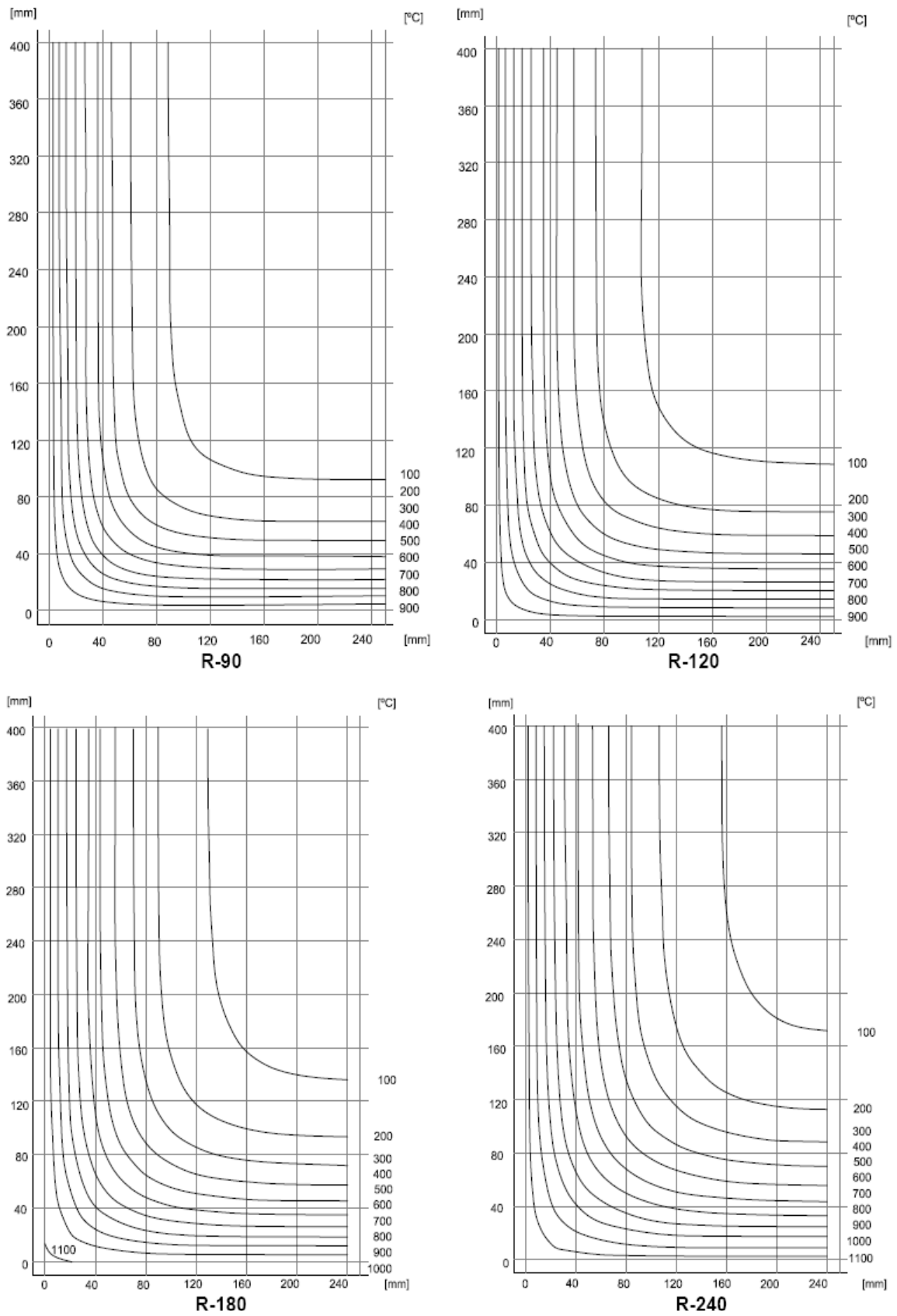
Figura C.5. Isotermas para cuartos de sección de 800 x 500 mm expuestos por ambas caras
